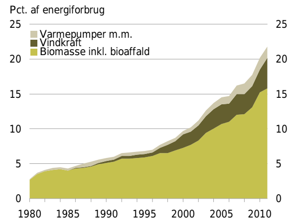
Figur 4.7 Vedvarende energi som andel af energiforbruget, 1980-2011
